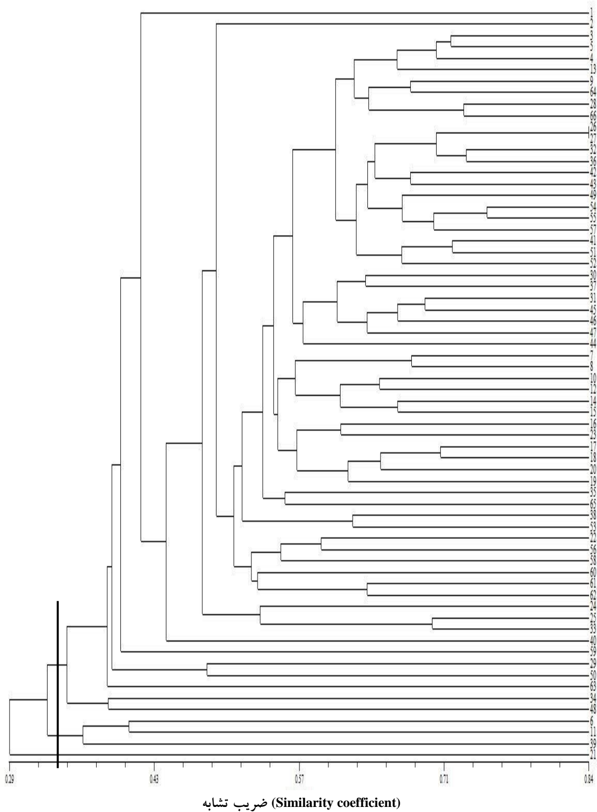
شکل ۱- دندروگرام مربوط به گروه‌بندی ۶۶ فرد شیرین‌بیان با استفاده از داده‌های ISSR Figure 1. UPGMA cluster analysis of different 66 individuals of G. glabra based on ISSR data matrix
