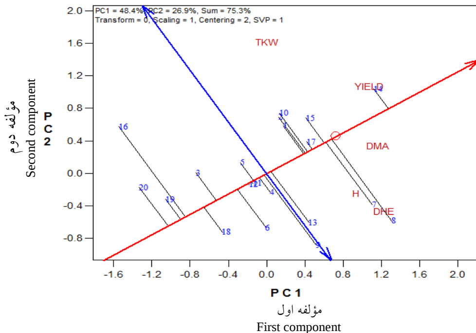
شکل ۲- بای پلات ۲۰ ژنوتیپ گندم از نظر صفات مختلف
