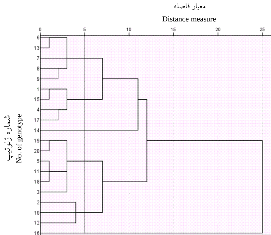
شکل ۱- تجزیه خوشه‌ای ژنوتیپ‌های گندم نان برای صفات مختلف به روش Ward
