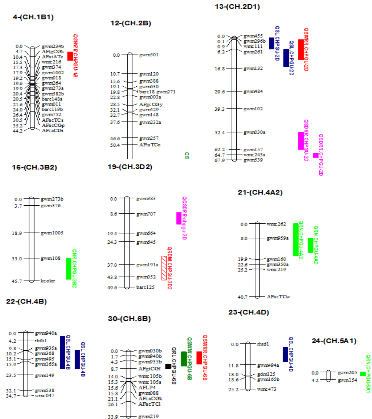
شکل ۲- مکان QTL‌های شناسایی شده برای صفات گیاهچه‌ای در جمعیت اینبرد لاین نوترکیب؛ کروموزوم (CH) و موقعیت کیوتی‌ال-های صفات تعداد ریشه‌چه (RN)، وزن خشک ساقه‌چه (SDW)، وزن خشک ریشه‌چه (RDW) و نسبت وزن خشک ساقه‌چه به وزن خشک ریشه‌چه (SDRR)، نسبت وزن تر ساقه‌چه به وزن تر ریشه‌چه (SWRR)، طول ساقه‌چه (SL)، طول ریشه‌چه (RL) و وزن تر ساقه‌چه (SWW).
