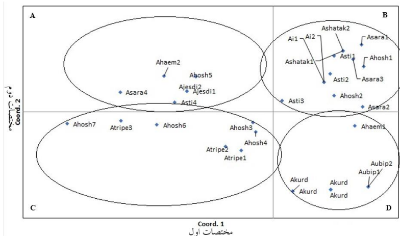
شکل ۳- تجزیه به مختصات اصلی اکوتیپ‌های جنس Allium بر اساس داده‌های ژنتیکی ISSR
