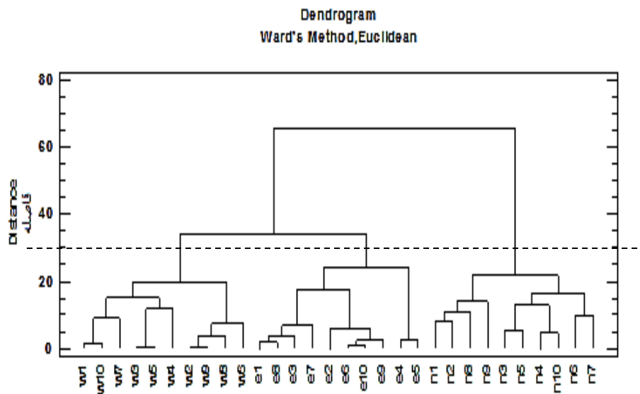
شکل ۱- دندروگرام حاصل از تجزیه کلاستر به روش Ward بر اساس صفات مورفولوژیکی بررسی شده
